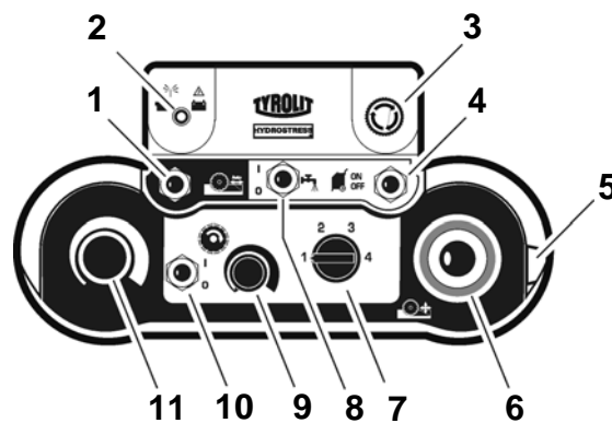
Fig. 4-2 Télécommande radio
