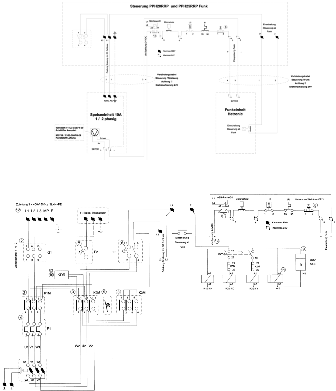
Fig. 3-3 Schéma électrique
