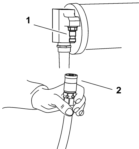
Fig. 4-9 Raccord d'eau
