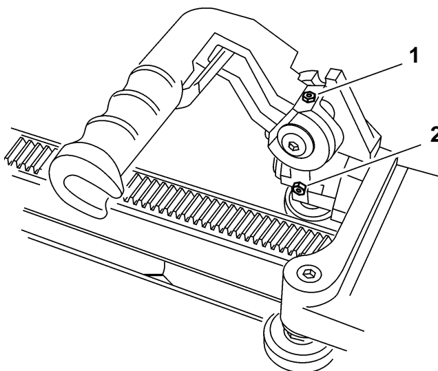
Fig. 6-1 Graisseurs
